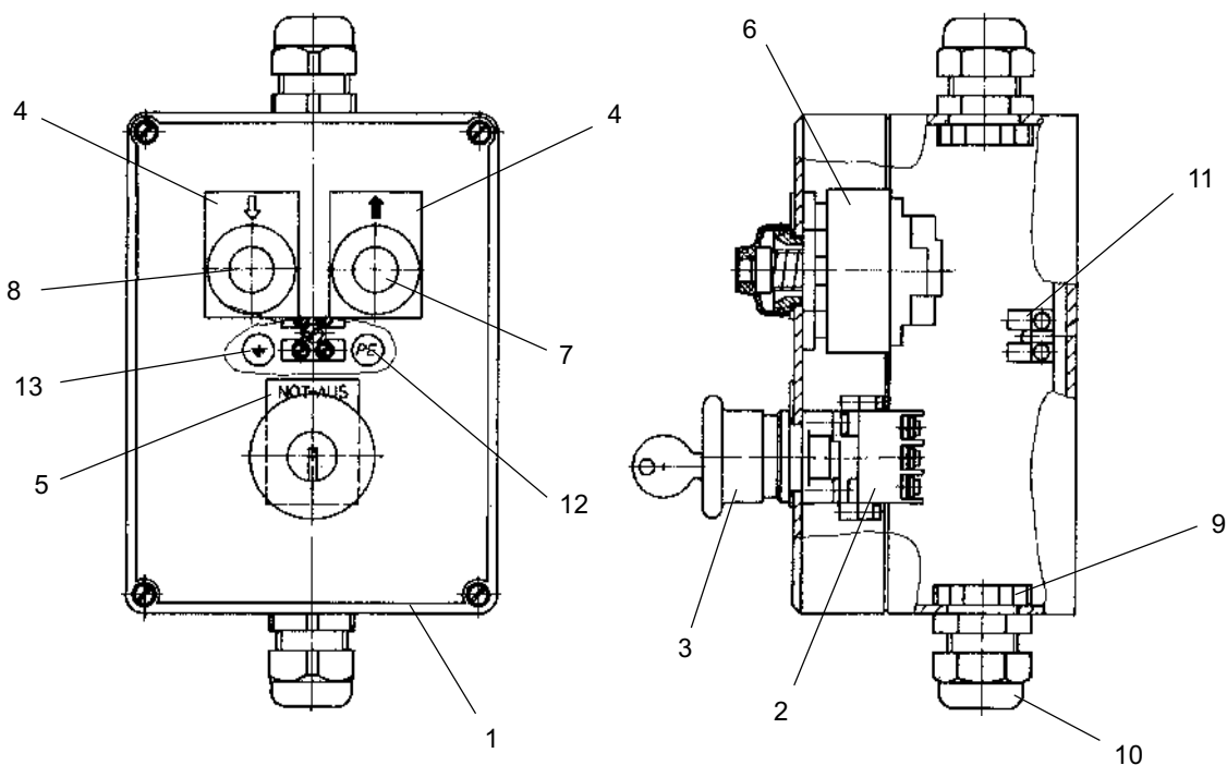
Abb. 18: Wandschalter
