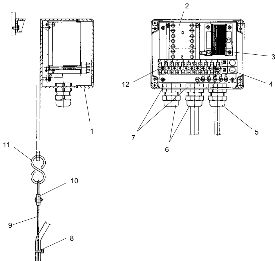
Abb. 15: Schützsteuerung
